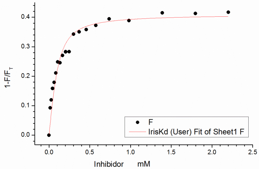
Gráfico 2_C pH 9.0
