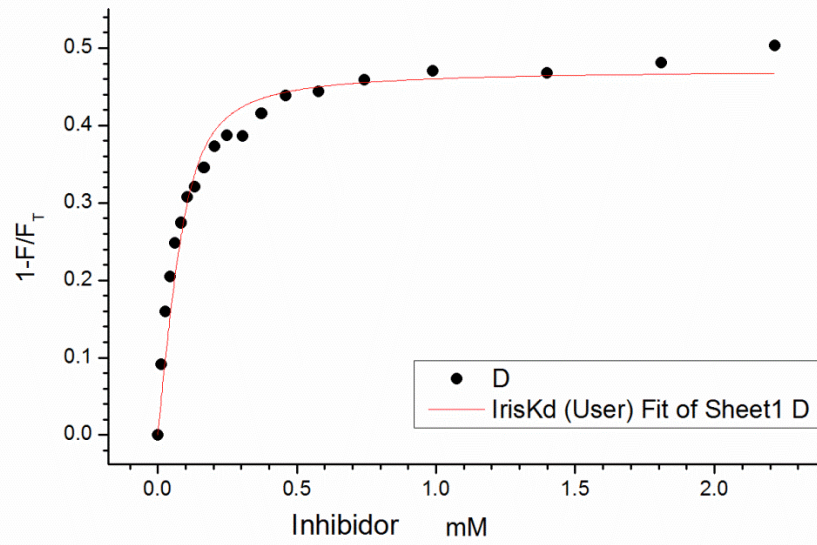
Gráfico 2_B pH 9.0
