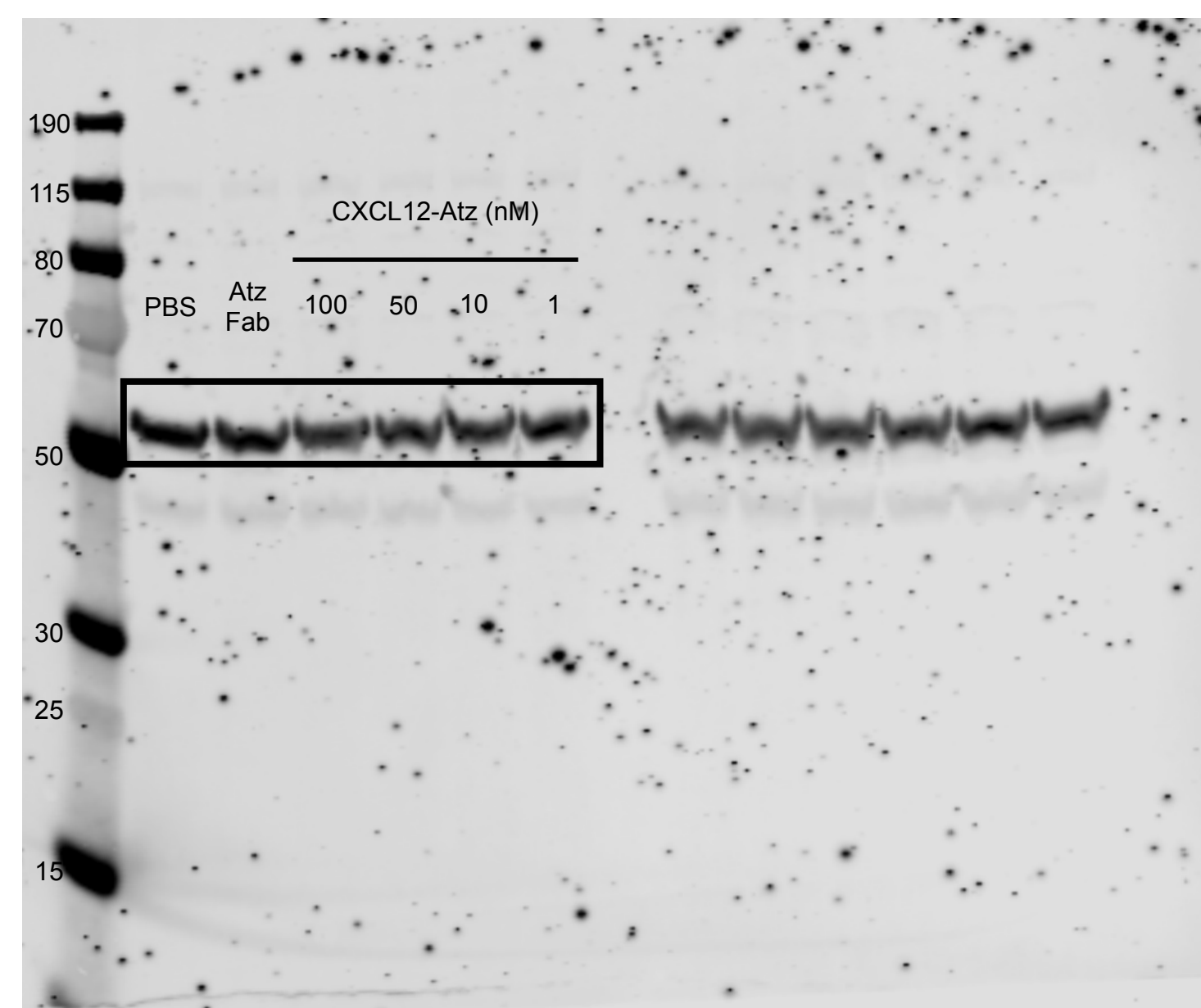
Tubulin blot
