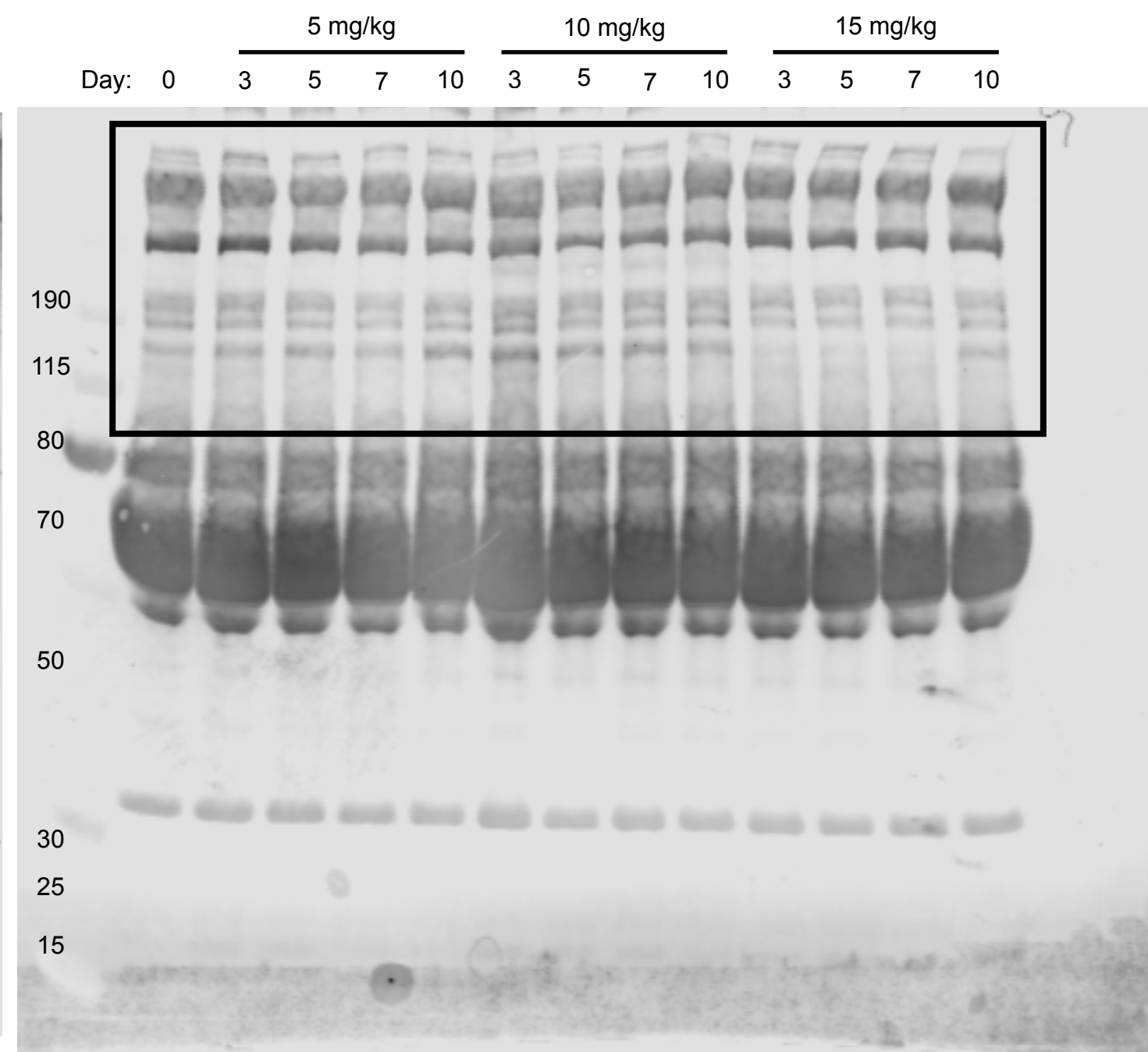
Tubulin blot
