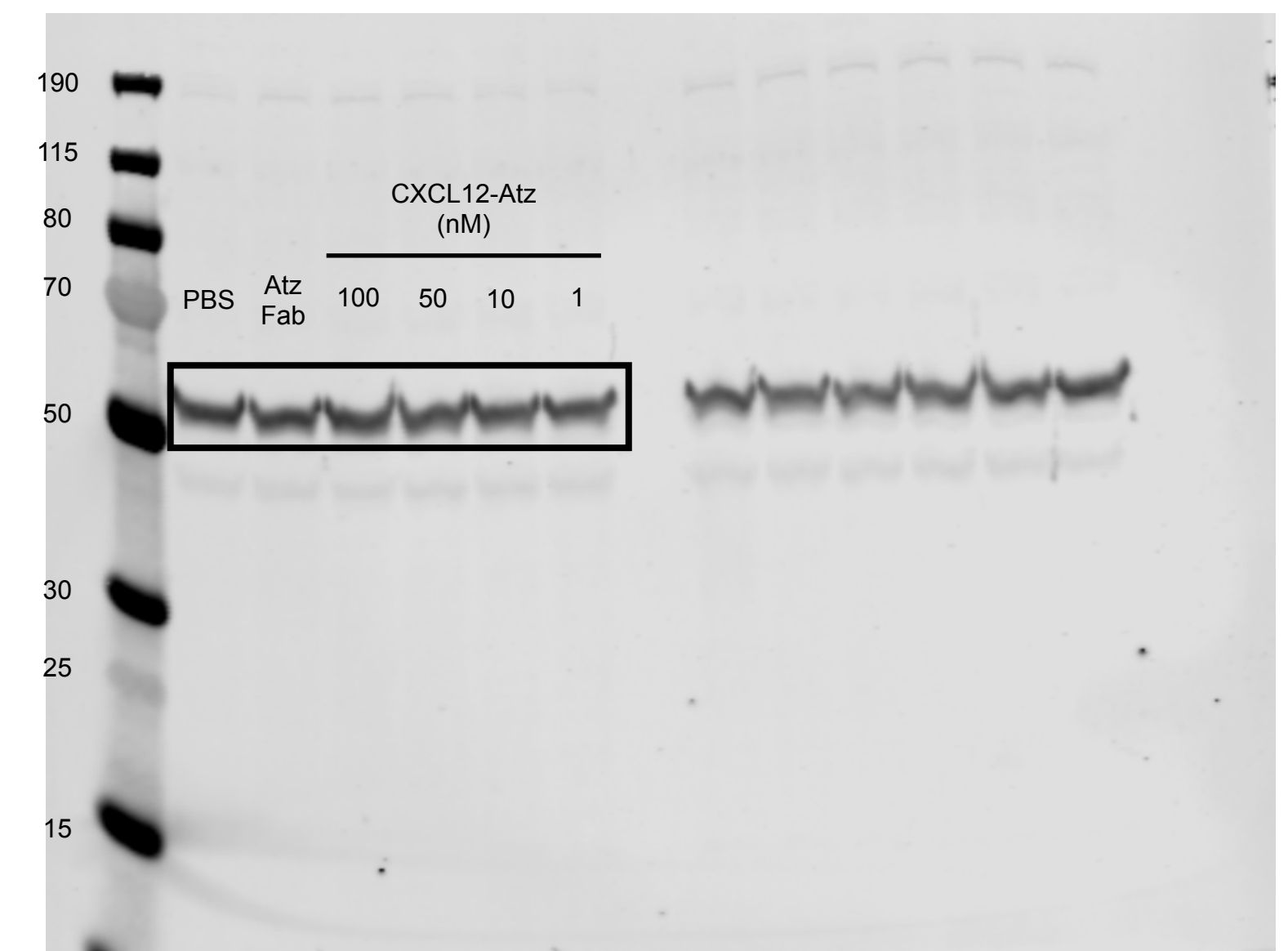
Tubulin blot
