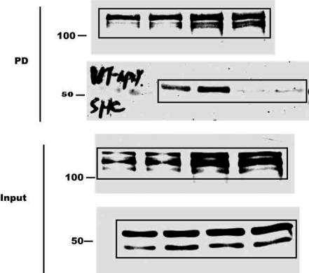
2J: MOLM13
