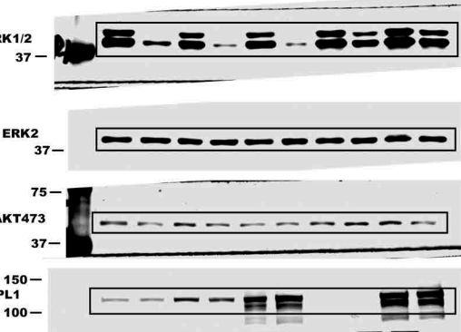
2I: MOLM13
