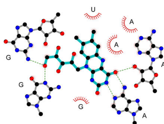
FMN riboswitch (RNA)
